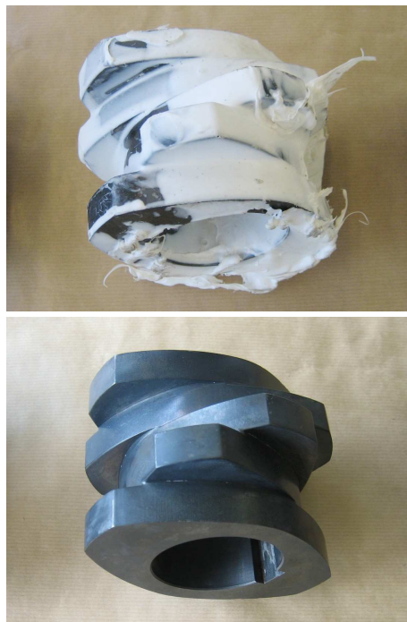
Segment de vis sans fin avant et après le nettoyage
